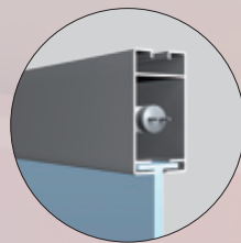
Profil eckig: Profilgröße 76 x 40 mm
